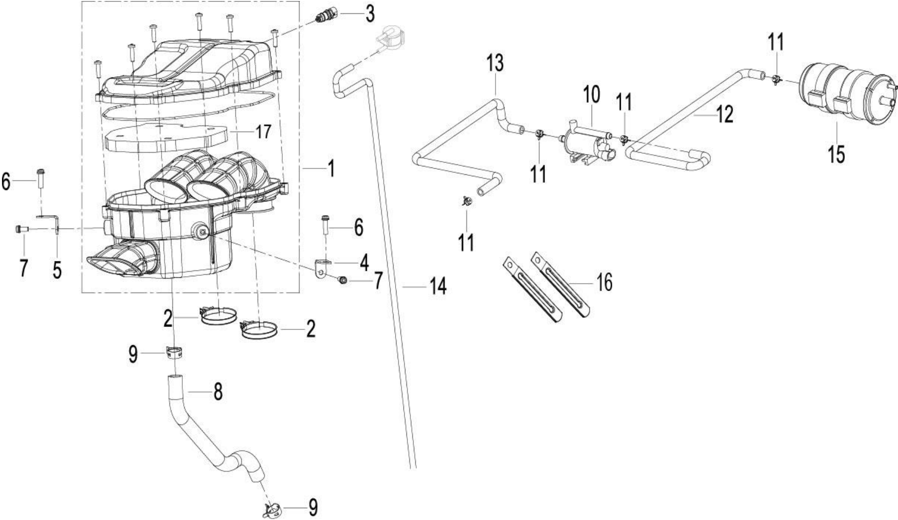
F06 空滤器 AIR CLEANER ASSY.
